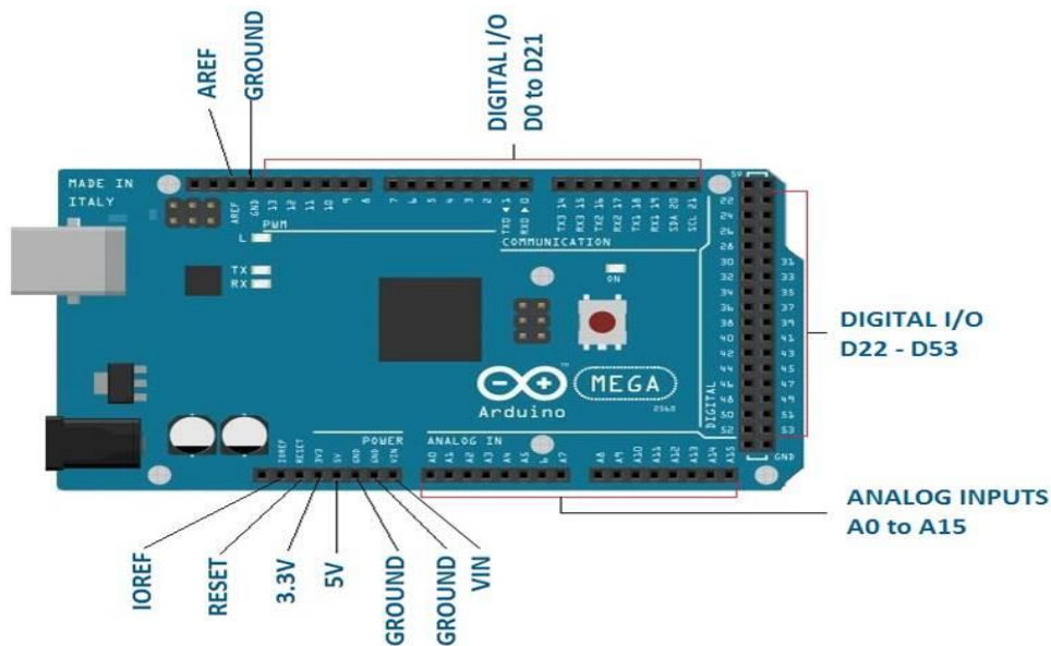
圖 6、Arduino Mega 2560
