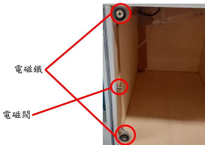
圖 11、電磁閥及電磁鐵
