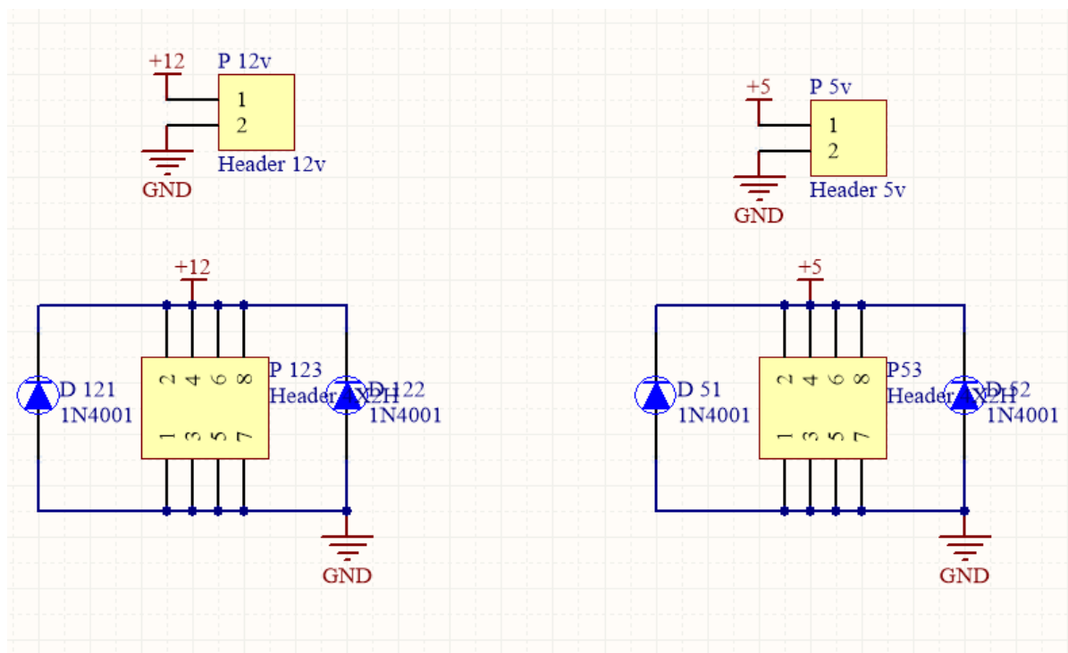
圖 17、電路圖
