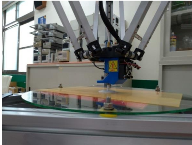
圖 16、3D 列印印製過程
